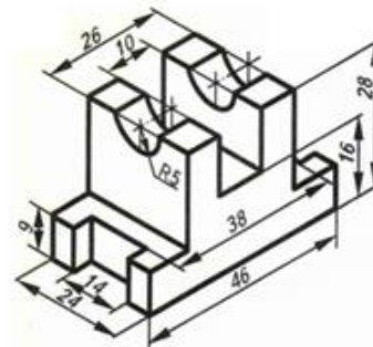
АКСОНОМЕТРИЧНА ПРОЕКЦІЯ
